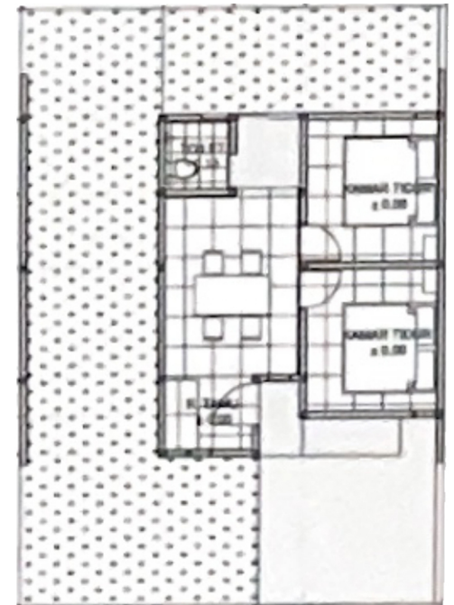
DENAH RUMAH TUMBUH TYPE 36 SEBELUM PENGEMBANGAN
