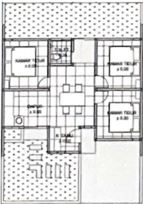
DENAH RUMAH TUMBUH TYPE 54 SESUDAH PENGEMBANGAN
