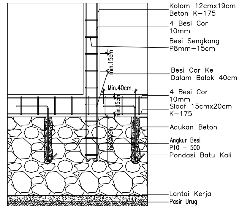
DETAIL SAMBUNGAN SLOOF-KOLOM 1 : 20
