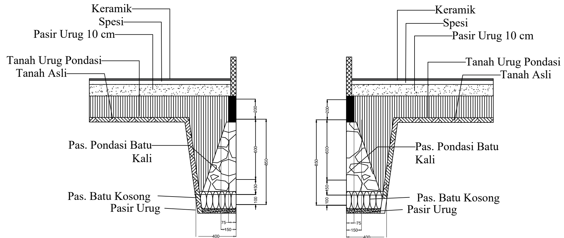
DETAIL PONDASI BATU KALI A 1 : 50
