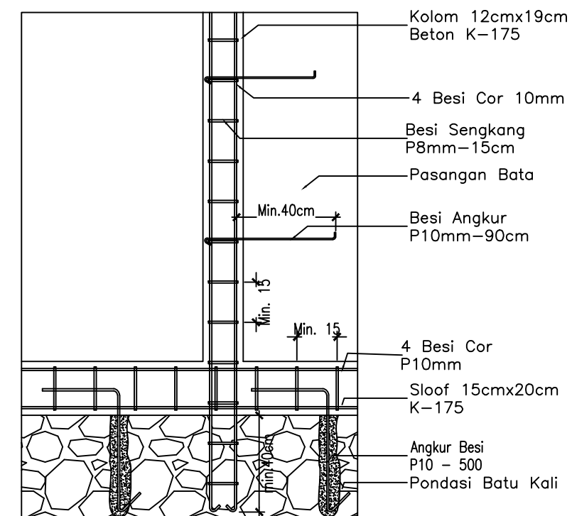
DETAIL SAMBUNGAN KOLOM-DINDING 1 : 20
